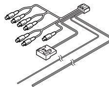
③ Câbles d'interconnexion (subwoofer, sortie de ligne, impulsion de vitesse, frein de stationnement, marche arrière, sortie de vidéo et connecteur de télécommande de direction) (16P) x 1
